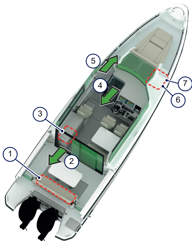
Figur 4.21 - Säkerhetsutrustning och nödutgångar
