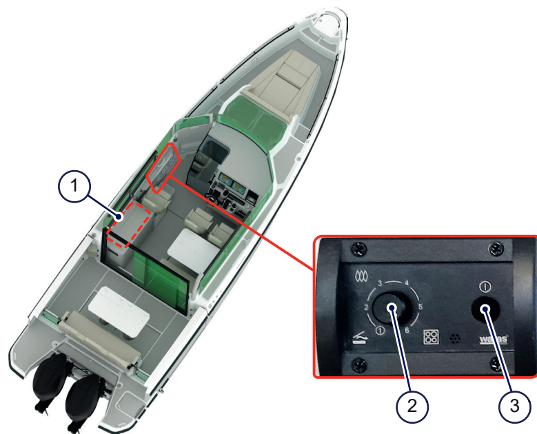
Figur 4.18 - Spishällens kontrollpanel
