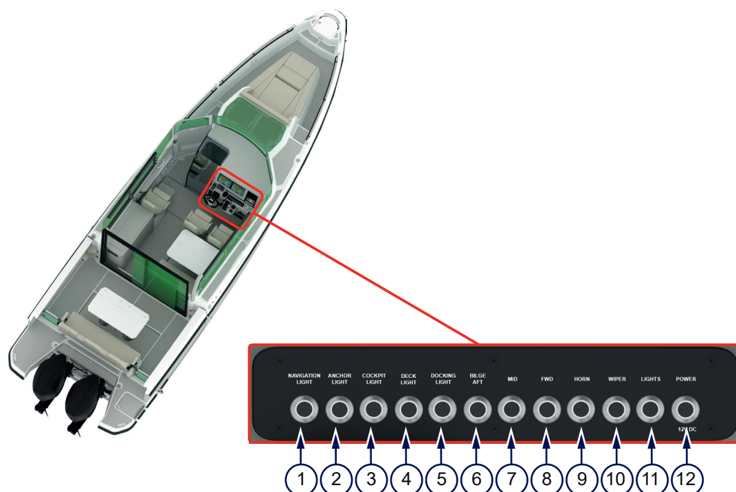
Figur 4.9 - Reglage på kontrollpanelen för navigation och belysning
