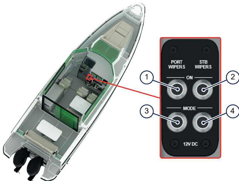
Figur 4.11 - Torkarkontrollpanel
