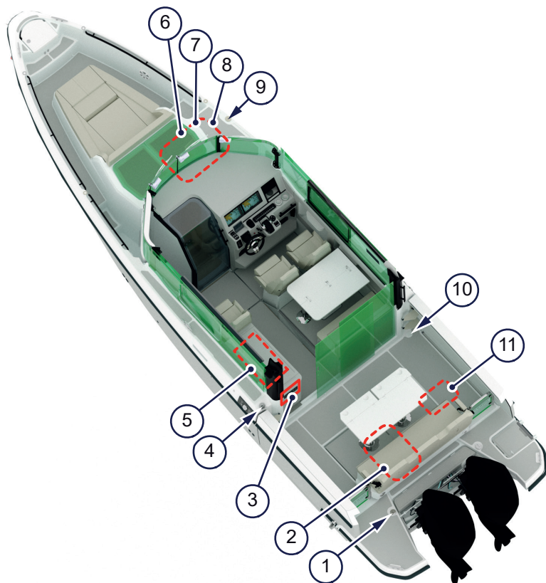
Figur 5.6 - Färsk-, grå- och svartvattensystem
