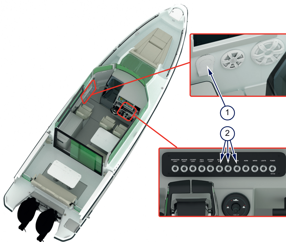
Figur 5.5 - Manuell länsypump och de automatiska länsypumparnas reglage
