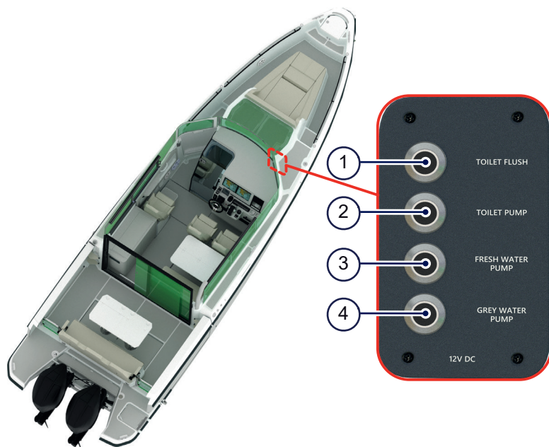
Figur 4.12 - Toalettutrymmets kontrollpanel
