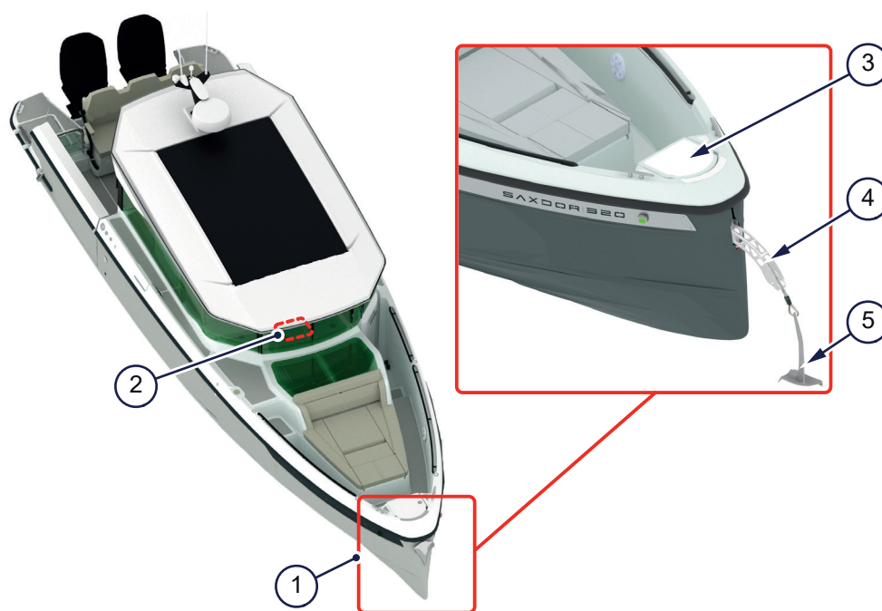
Figur 5.8 - Ankarsystem
