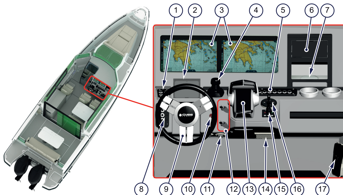
Figur 4.8 - Förarplatsens reglage
