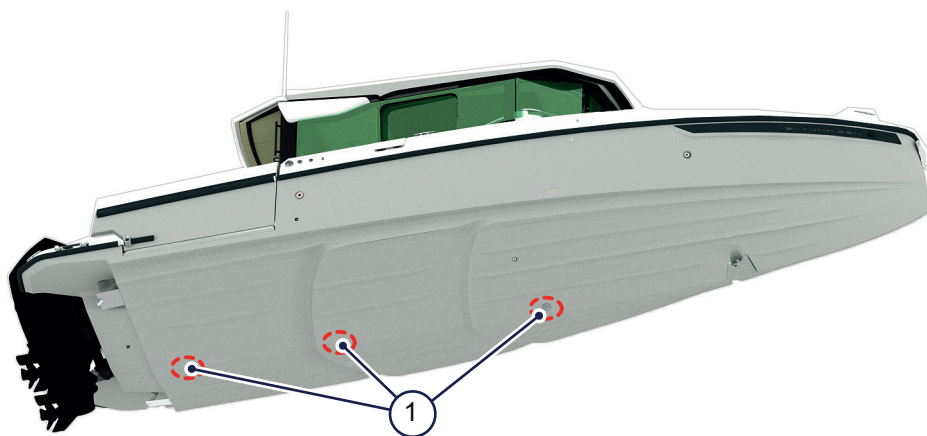
Figur 5.4 - Automatiska länsumpar
