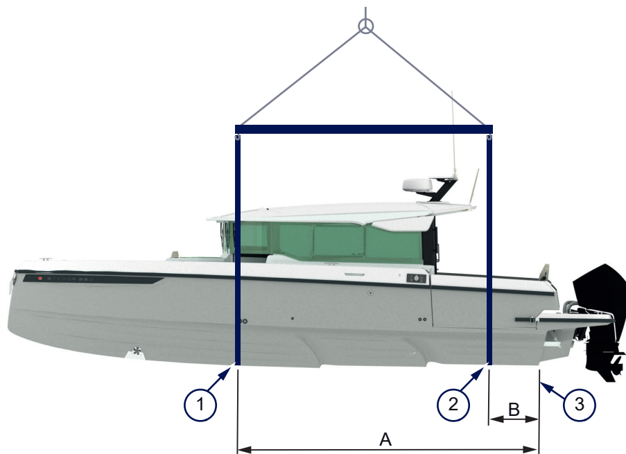
Figur 4.25 - Lyftpunkter
