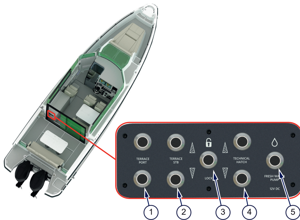
Figur 4.13 - Terrasskontrollpanel
