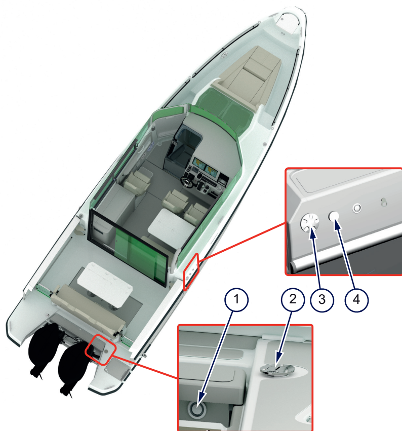
Figur 5.3 - Bränslesystem
