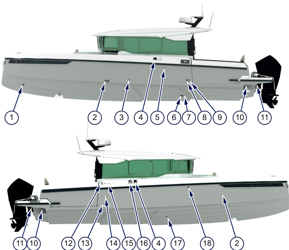
Figur 4.26 - Skrovöppningar
