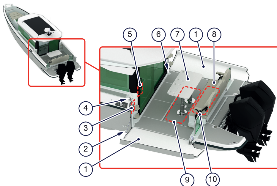
Figur 4.5 - Akterdäck
