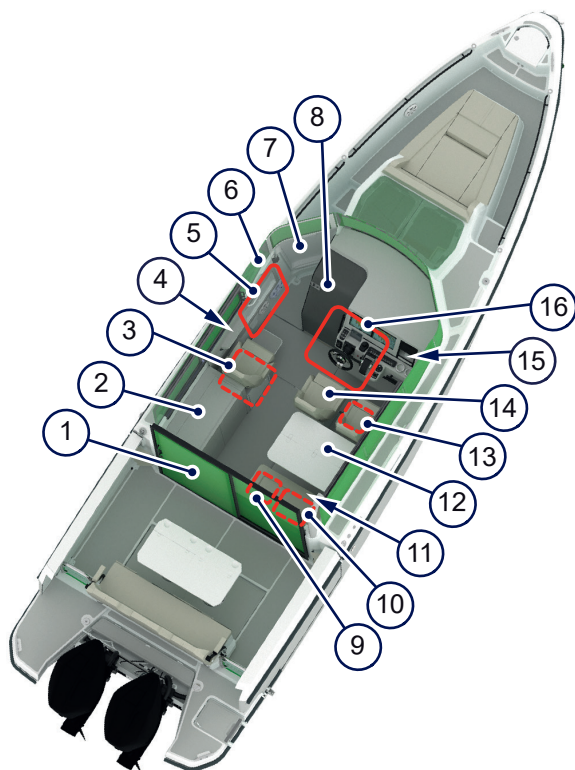
Figur 4.4 - Huvudhytt
