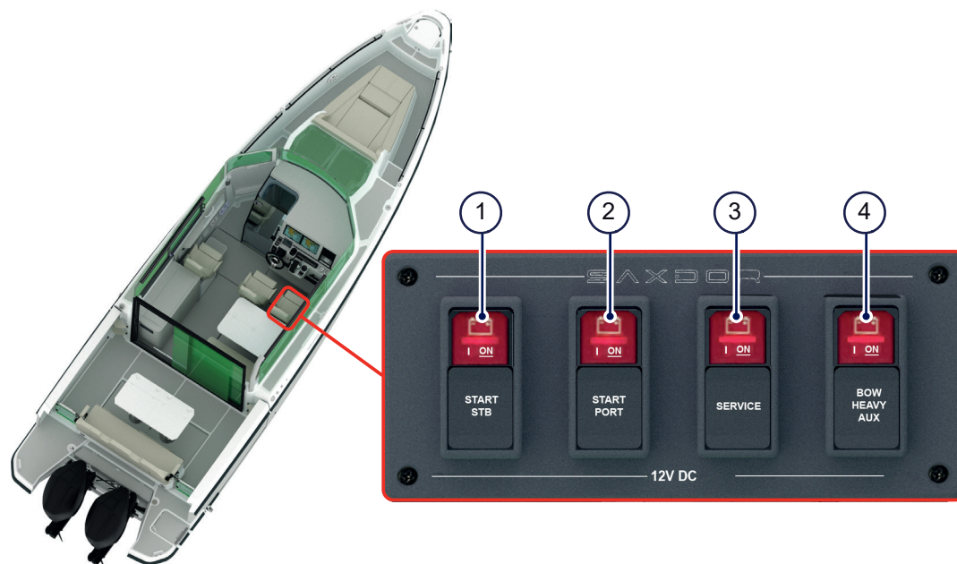
Figur 4.16 - Batterikontrollpanel
