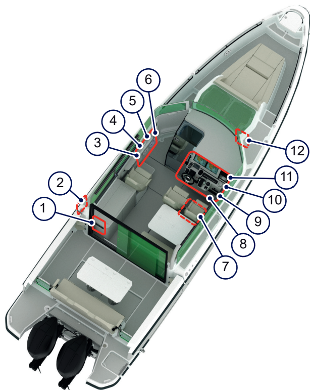
Figur 4.7 - Placering av användarreglage
