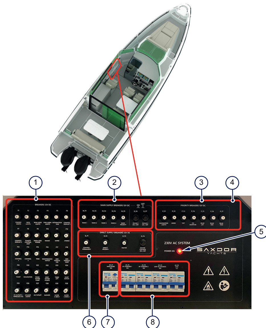
Figur 4.15 - Främre hyttens säkringspanel
