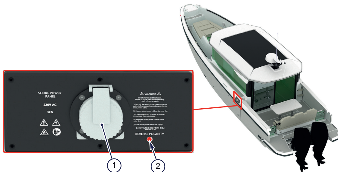
Figur 4.17 - Landströmspanel
