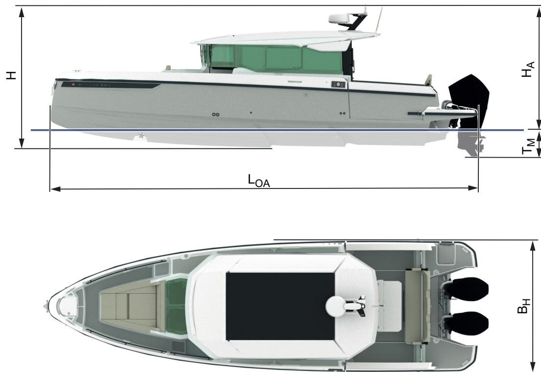
Figur 8.1 - Saxdor 320 GTC dimensioner
