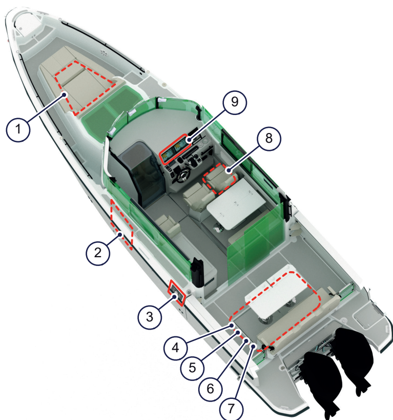
Figur 5.1 - Elsystem
