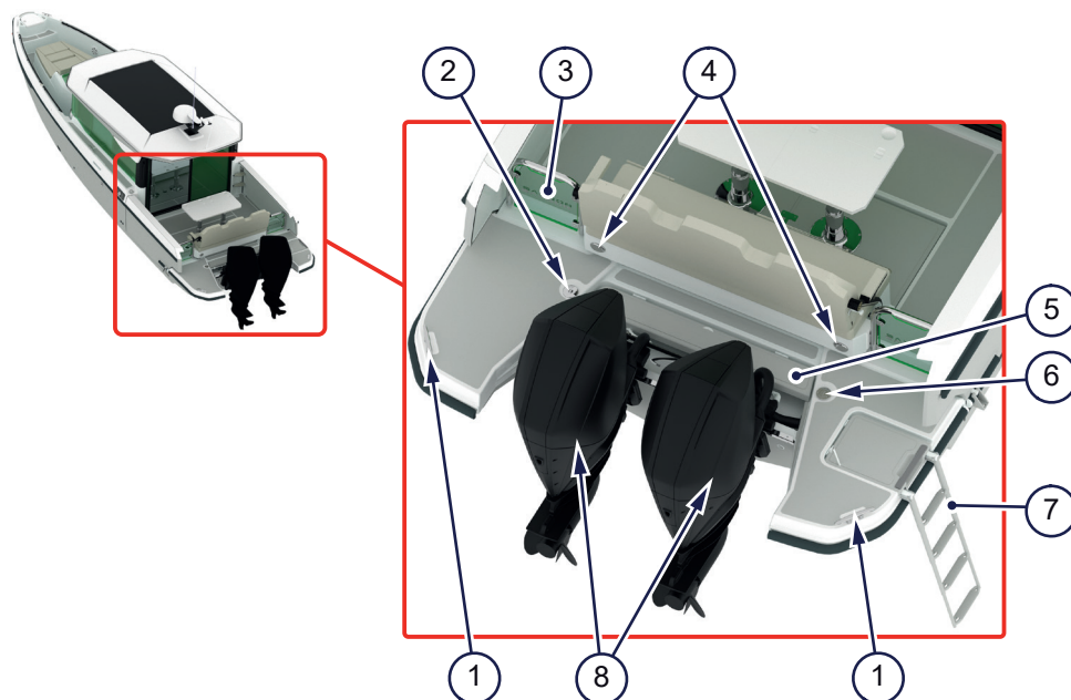
Figur 4.6 - Badplattform
